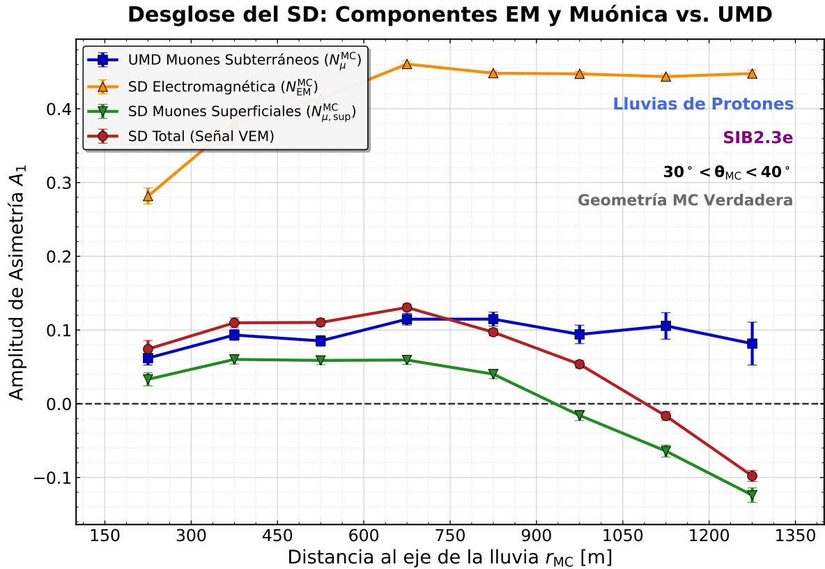
Figura 6.4: Desglose de la asimetría azimutal para las componentes inyectadas a nivel del suelo frente a la respuesta del detector subterráneo ( 30^\circ \leq \theta < 40^\circ ). La asimetría electromagnética del SD (naranja) exhibe un comportamiento marcadamente positivo acoplado a la evolución longitudinal. En contraste, los muones superficiales registrados por el SD (verde) presentan una pronunciada asimetría negativa. La combinación destructiva de estas dos poblaciones genera la inestabilidad de la señal total en superficie, validando al mismo tiempo la necesidad del blindaje del UMD (azul) para aislar la direccionalidad muónica pura de la cascada.
